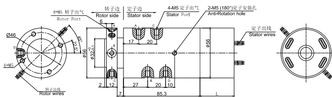
DA PH400F-01 尺寸图
