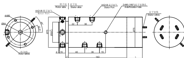
DA PH400F-03 尺寸图
