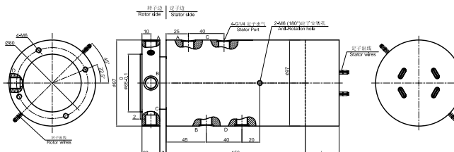
DA PH400F-03 尺寸图
