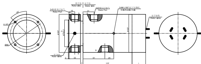
DAIPH200F-05 尺寸图
