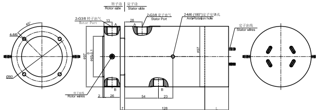
DAIPH200F-05 尺寸图
