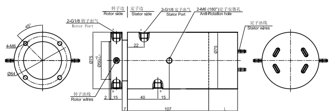
DAPH200F-02 尺寸图
