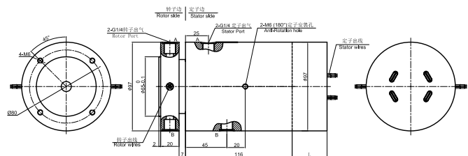
DAPH200F-03 尺寸图
